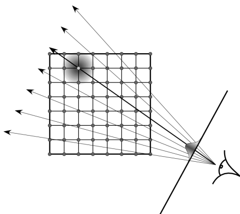
FIG. 2.10 – Discrétisation implicite de l'intégrale de rendu volumique par la technique du "splatting". La contribution de chaque voxel à l'image finale est calculée par projection. L'empreinte ("footprint" en anglais) du voxel projeté (gris clair) sur l'image dépend d'un noyau de convolution (gaussien dans notre cas) appliqué avant projection.
