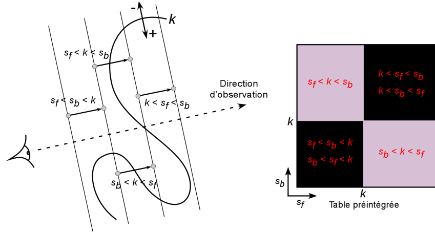
FIG. 4.6 – Cas particulier de table préintégrée pour la visualisation de surfaces d'isovaleur non polygonales. La surface d'isovaleur en gras est échantillonnée avec quatre tranches orthogonales à la direction d'observation. En fonction des valeurs du couple \{s_f, s_b\} par rapport à l'isovaleur k , quatre cas distincts sont envisageables. Les rectangles noir et gris clair dans la table ont respectivement une opacité nulle et maximale.
