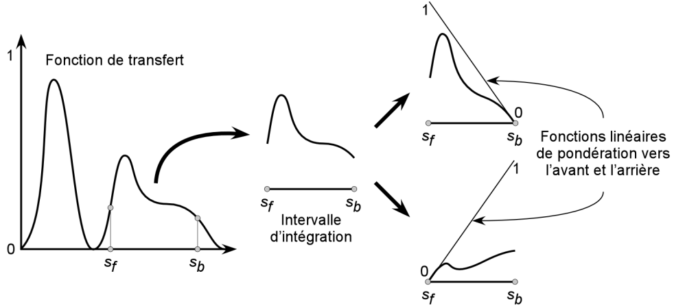
FIG. 3.13 – Principe de l'intégration pondérée dans la technique d' illumination préintégré interpolée . La contribution de l'émission des sous-segment dans la table classique est multipliée par une fonction rampe orientée selon le cas vers l'avant ou l'arrière du segment (modifié d'après [LUM E.B. et al., 2004]).
