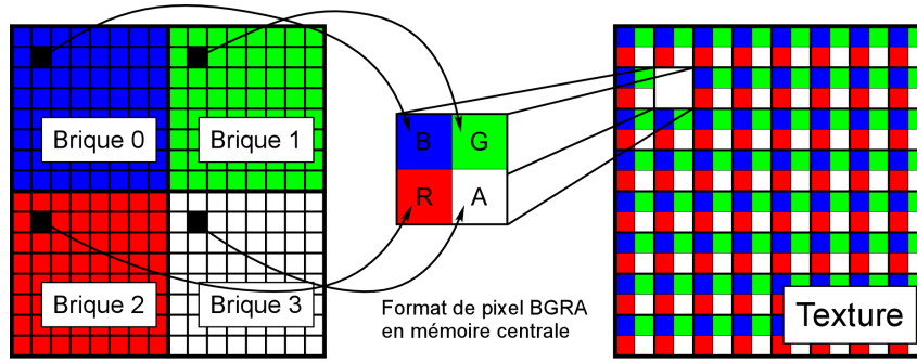
FIG. 6.10 – Principe d’entrelacement des valeurs scalaires de quatre briques dans une seule texture GL_BGRA (stockée dans un format interne GL_RGBA8 ).
