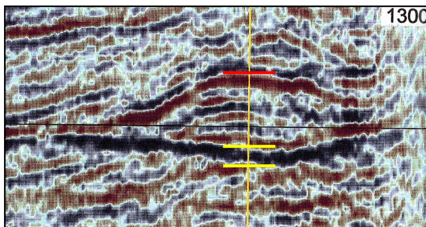
FIG. 1.6 — Anomalie positive de l'amplitude sismique, ou " bright spot ", correspondant à un contact eau-gaz dans un réservoir offshore du delta du Nil (Égypte). Les marqueurs jaunes encadrent le " bright spot " et le marqueur rouge correspond au toit du gaz (d'après [BROWN A.R., 2004]).
