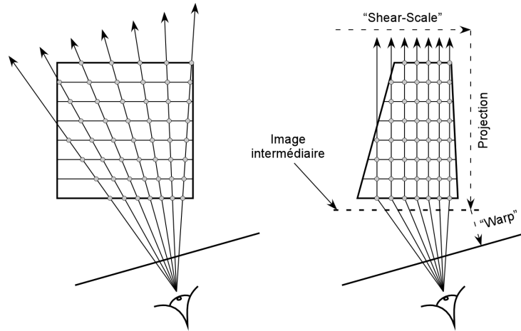
FIG. 2.11 – Discretisation implicite de l'intégrale de rendu volumique par la technique du "shear-warp". Après cisaillement-homothétie ("shear-scale") du volume, la composition est calculée par projection sur une image intermédiaire distordue puis plaquage ("warp") sur l'image finale.
