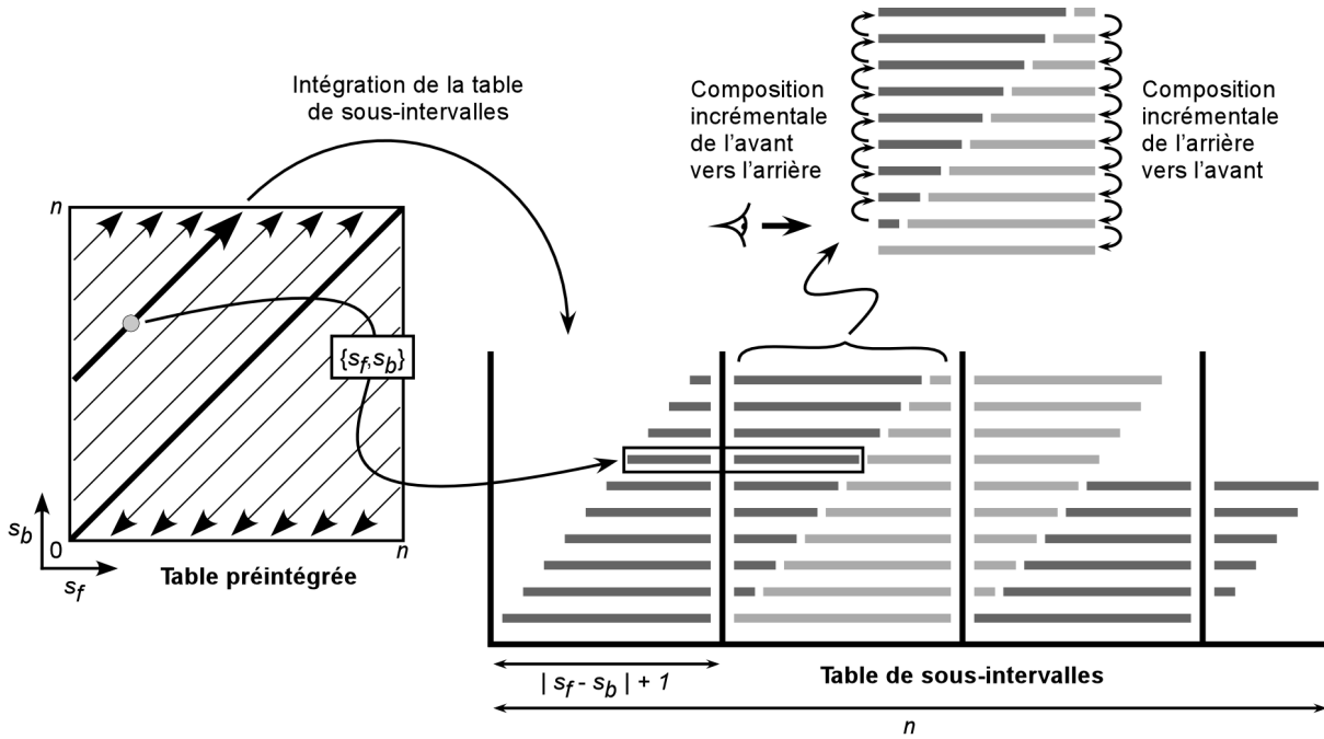
FIG. 3.11 – Préintégration de la fonction de transfert à l'aide de l'algorithme des sous-intervalles incrémentaux . Le remplissage de la table préintégrée est effectué diagonale par diagonale, formant ainsi des groupes de segments [s_f, s_b] dont le nombre de sous-segments est identique. Pour chaque diagonale, une table de sous-intervalles est intégrée incrémentalement en un temps O(n) où n est la taille de la fonction de transfert. Les résultats intermédiaires sont stockés et, pour tout couple \{s_f, s_b\} dans la diagonale, les deux sous-intervalles correspondants sont composés. Pour une table de taille n \times n , le calcul des 2n - 1 diagonales se fait donc en un temps O(n^2) (modifié d'après [LUM E.B. et al. , 2004]).
