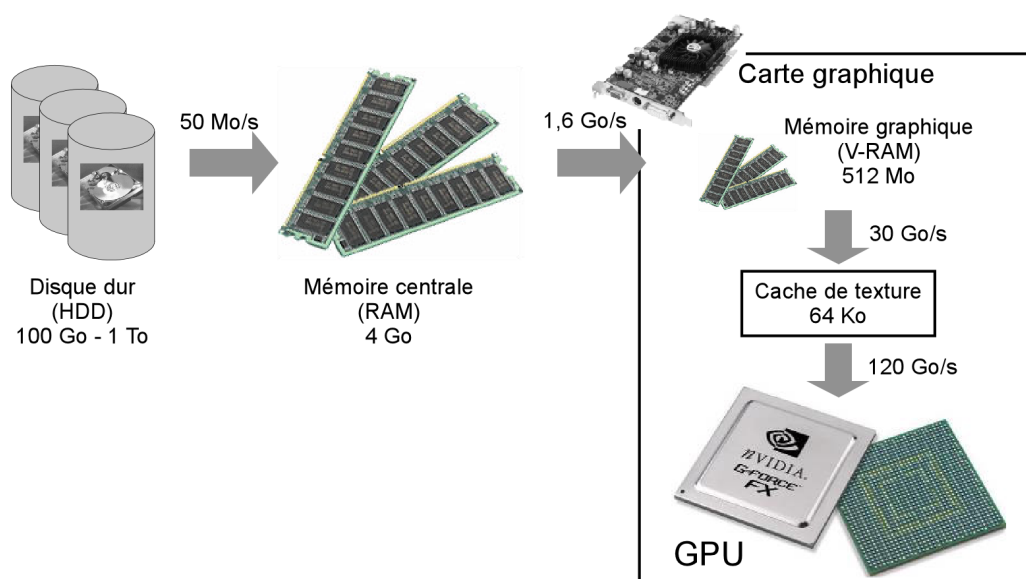
FIG. 5.1 – Hiérarchies de mémoire comparées du processeur central (haut) et du processeur graphique (bas). La notion de cache est généralisée, chaque niveau jouant le rôle de cache du niveau suivant. Les bandes passantes sont données à titre indicatif pour un accès unidirectionnel en lecture aux données (obtenues à partir de SiSoftware Sandra 2007 [SISOFTWARE SANDRA 2007, -]).
